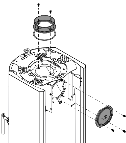
Fig. 15: Smontaggio del coperchio e della presa della canna fumaria
