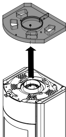
Fig. 11: Rimozione del coperchio
