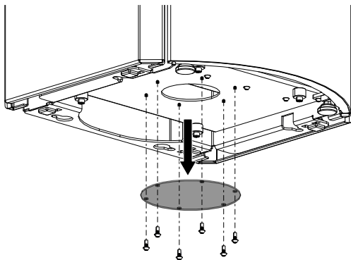
Fig. 33: Rimozione della piastra di tenuta dal basso
