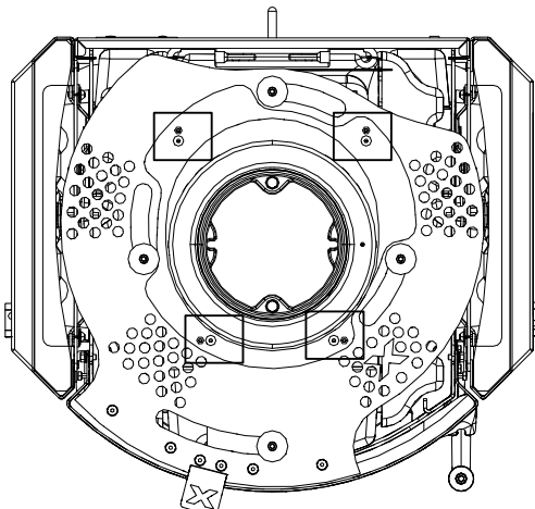
Fig. 42: Ventola dall'alto
